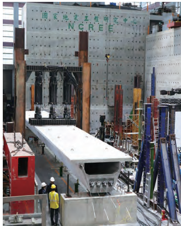
超高性能混凝土預力梁 (U258) 簡支單向加載試驗
