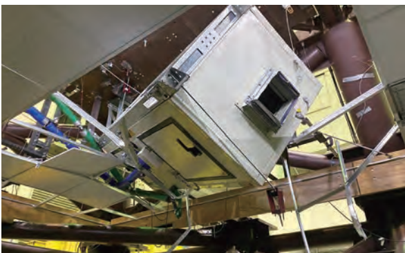
與日韓合作之實驗證實耐震不佳之懸吊設備易危害生命安全
